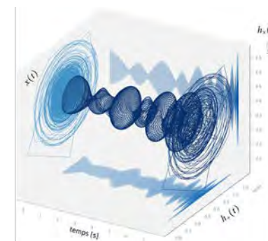
^ Onde gravitationnelle x(t) et ses deux composantes (aussi appelées polarisations) h+(t) et h x(t) émise par un système binaire de trous noirs en coalescence.
